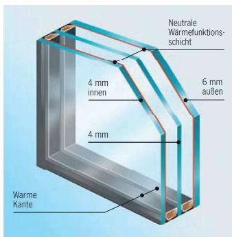
3-Scheiben-Wärmeschutzverglasung mit Edelgasfüllung Ug 0.7 Schalldämmung 36 dB Triple vitrage thermo-isolant avec remplissage de gaz rare Ug 0.7 Isolation phonique 36 dB
