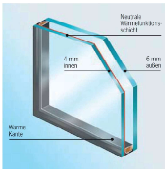
2-Scheiben-Wärmeschutzverglasung mit Edelgasfüllung Ug 1.1 Schalldämmung 36 dB Double vitrage thermo-isolant avec remplissage de gaz rare Ug 1.1 Isolation phonique 36 dB
