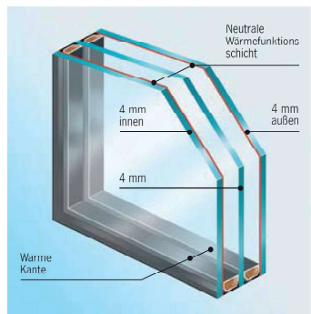
3-Scheiben-Wärmeschutzverglasung mit Edelgasfüllung Ug 0.6 Schalldämmung 32 dB Triple vitrage thermo-isolant avec remplissage de gaz rare Ug 0.6 Isolation phonique 32 dB
