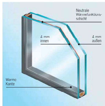
2-Scheiben-Wärmeschutzverglasung mit Edelgasfüllung Ug 1.1 Schalldämmung 30 dB Double vitrage thermo-isolant avec remplissage de gaz rare Ug 1.1 Isolation phonique 30 dB
