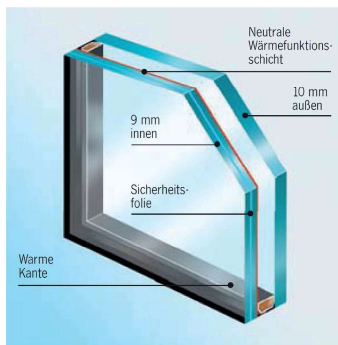
2-Scheiben-Wärmeschutzverglasung mit Edelgasfüllung Ug 1.1 Schalldämmung 44 dB Double vitrage thermo-isolant avec remplissage de gaz rare Ug 1.1 Isolation phonique 44 dB
