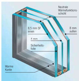
3-Scheiben-Wärmeschutzverglasung mit Edelgasfüllung Ug 0.7 Schalldämmung 42 dB Triple vitrage thermo-isolant avec remplissage de gaz rare Ug 0.7 Isolation phonique 42 dB
