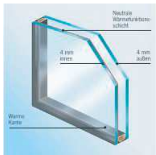
2-Scheiben-Wärmeschutzverglasung mit Edelgasfüllung Ug 1.1 Schalldämmung 30 dB*
