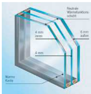
3-Scheiben-Wärmeschutzverglasung mit Edelgasfüllung Ug 0.7 Schalldämmung 36 dB*
