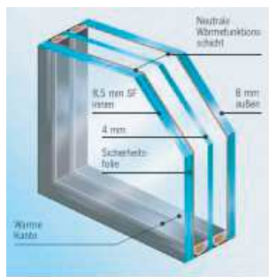
3-Scheiben-Wärmeschutzverglasung mit Edelgasfüllung Ug 0.7 Schalldämmung 42 dB*
