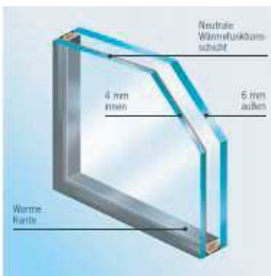
2-Scheiben-Wärmeschutzverglasung mit Edelgasfüllung Ug 1.1 Schalldämmung 36 dB*
