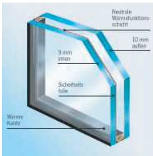
2-Scheiben-Wärmeschutzverglasung mit Edelgasfüllung Ug 1.1 Schalldämmung 44 dB*
