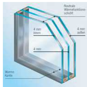
3-Scheiben-Wärmeschutzverglasung mit Edelgasfüllung Ug 0.6 Schalldämmung 32 dB*
